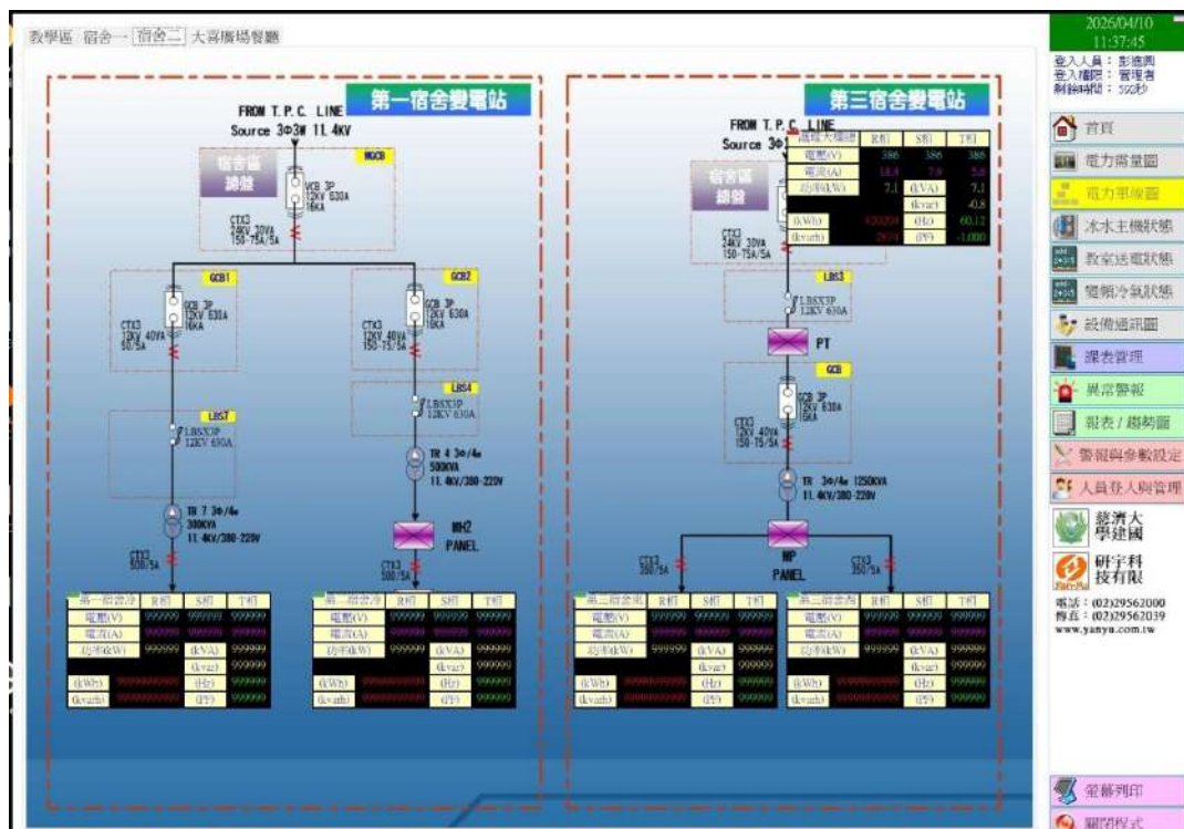
建國校區 EMS 系統設備時控
