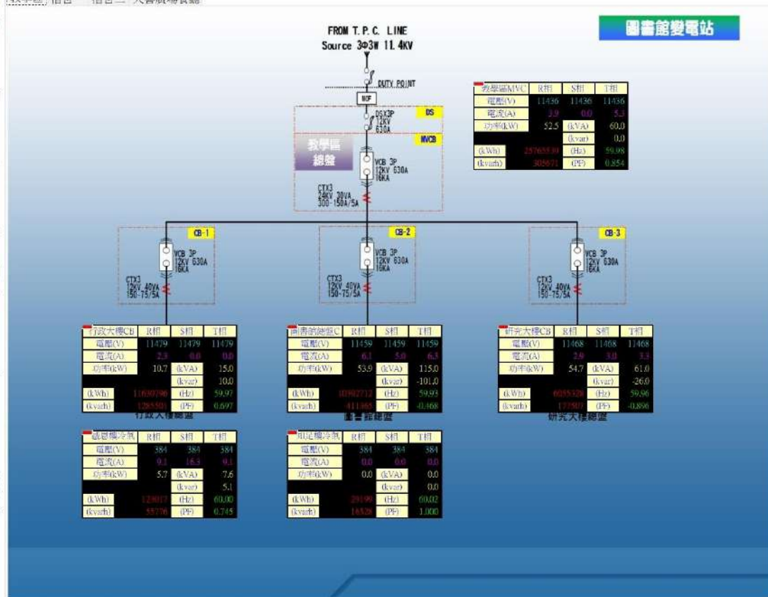
建國校區 EMS 系統宿舍區高壓系統
